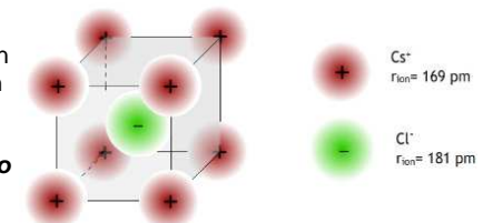
CsCl. Estructura cúbica centrada en el cuerpo. I.C. = 8
